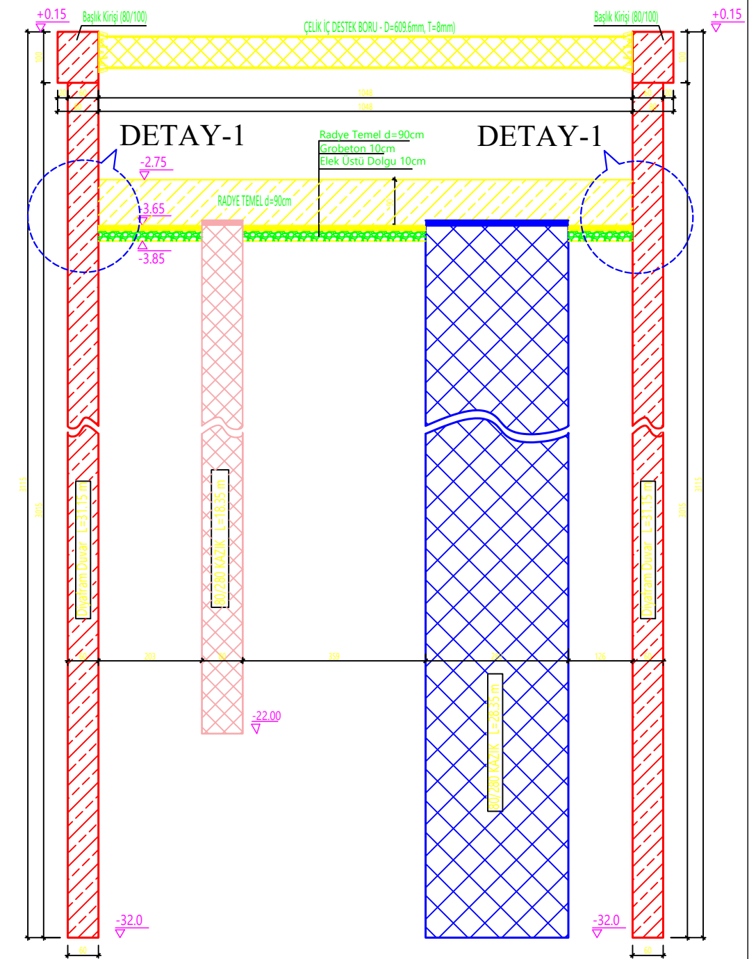
B-B KESITI (1/50)
